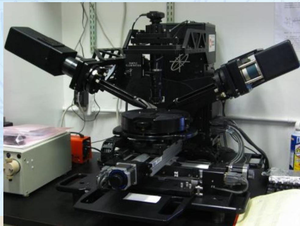
ЕЛИПСОМЕТЪР
